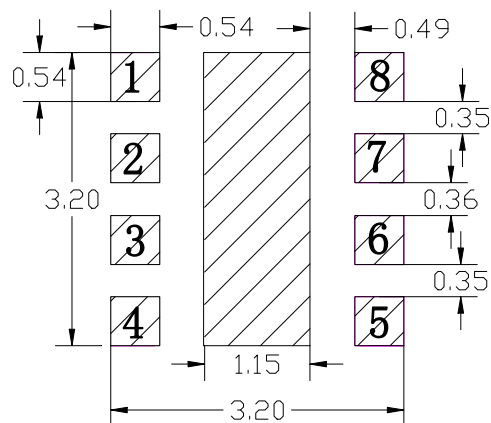
建议焊盘
