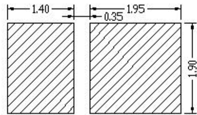
建议焊盘
