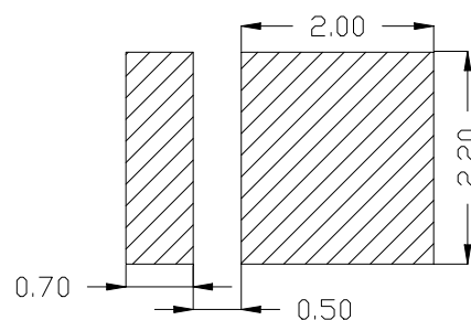
建议焊盘
